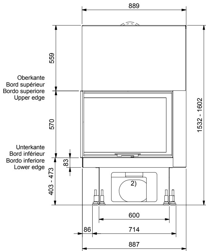
Frontansicht / Vue de face Vista frontale / Front view
