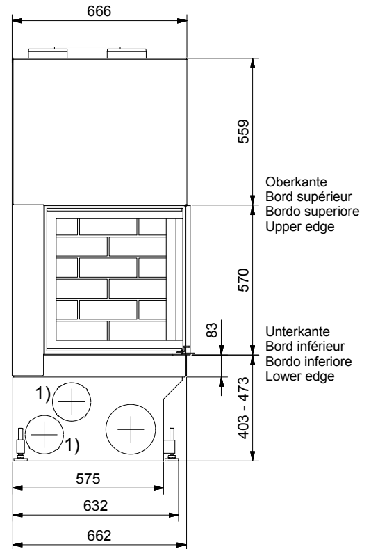
Seitenansicht / Vue de côté Vista laterale / Side view
