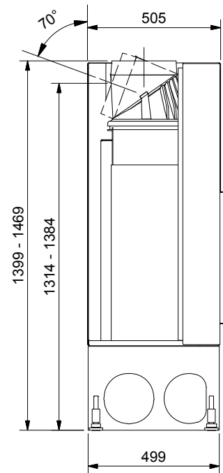
Seitenansicht / Vue de coté Vista laterale / Side view
